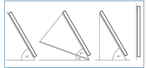
Possibilités de montage pour le capteur hybride SOLAERA:
